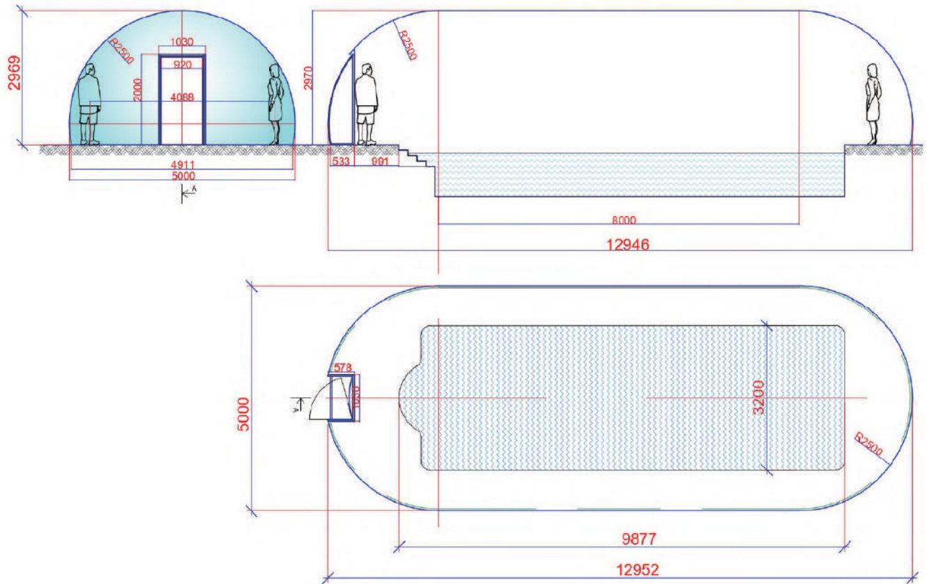
SECTION A-A
